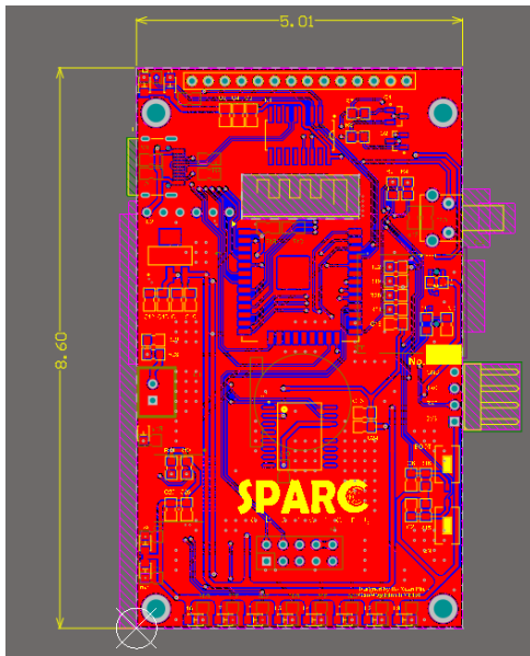
Hình 3.25 Lớp Top (Đường tín hiệu).
