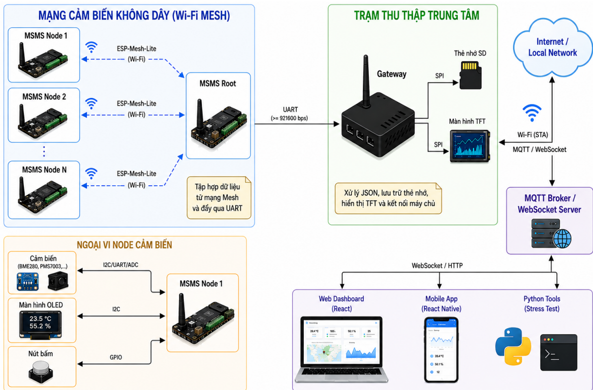
Hình 3.1 Cấu trúc tổng quan của hệ thống.
