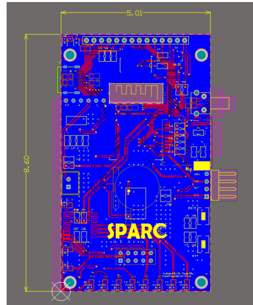
Hình 3.26 Lớp Bottom (Mặt dưới).
