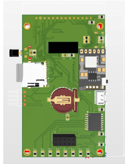
Hình 3.28 Mô hình 3D (Mặt dưới).
